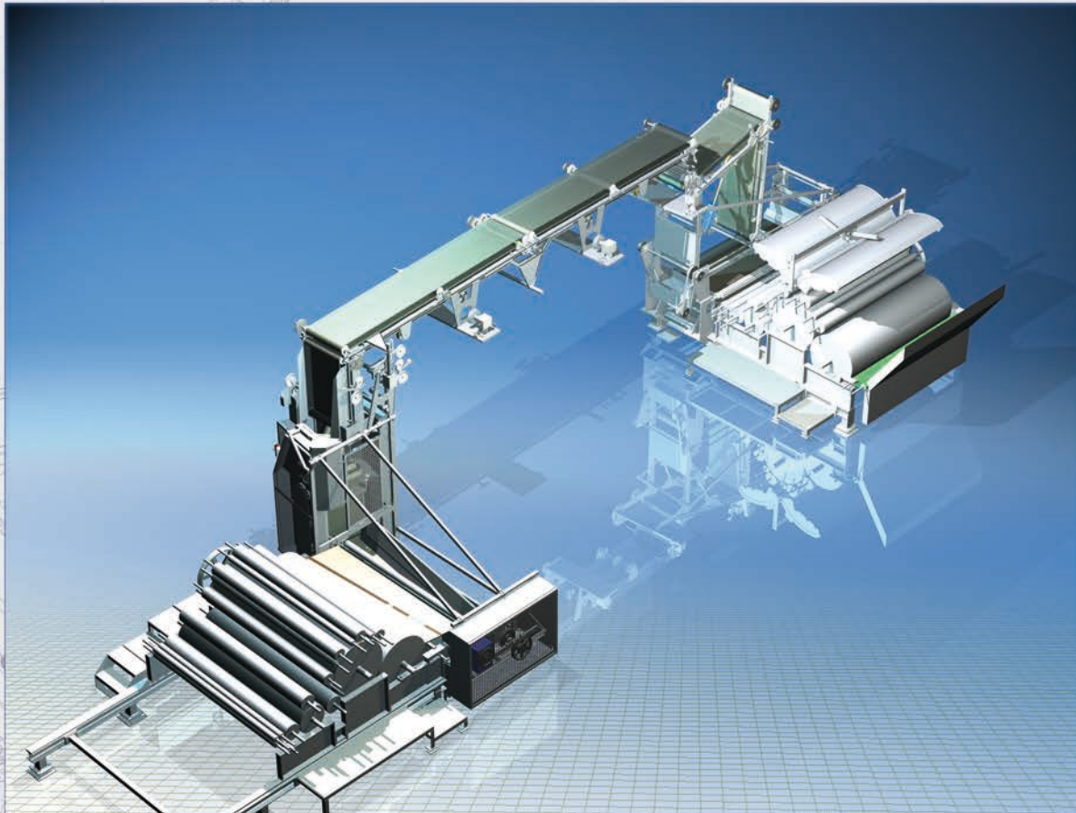
3D Konstruktion Kreuzvorleger
