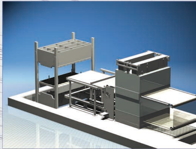
3D Konstruktion Umbau Fertigungsstraße
